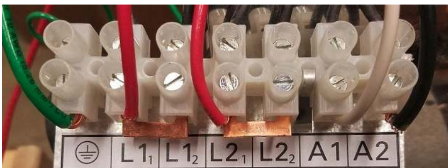
Heater Wiring
